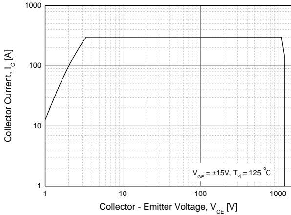
Fig. 7 RBSOA
