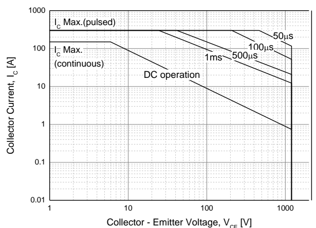
Fig. 6 SOA
